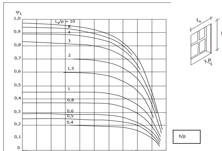
Grafico D.1.4.c – Fattore di riduzione apertura verticale \Psi_i
