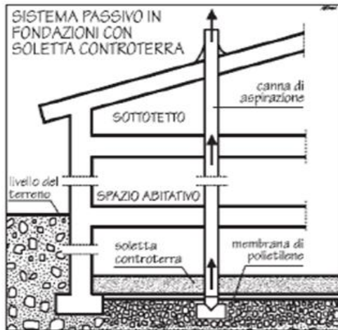
Fig.1 – Sistema passivo in fondazioni con soletta controterra; Fig 2 – Sistema passivo in fondazione con intercapedine.
