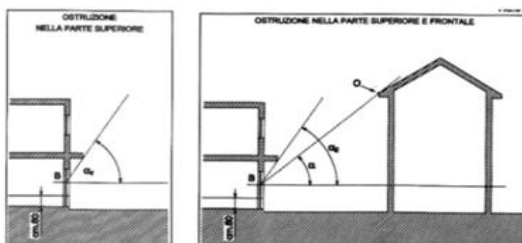
Figura 3 Parametri geometrici per ostruzione frontale e superiore
