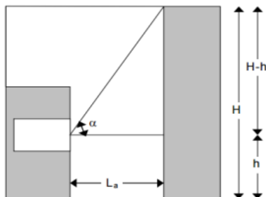
Figura 1 Valore del fattore finestra \varepsilon per ostruzioni poste di fronte alla finestra del locale considerato.
