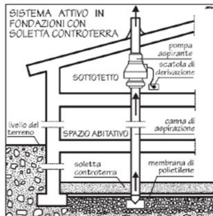
Fig.3 Sistema attivo.
