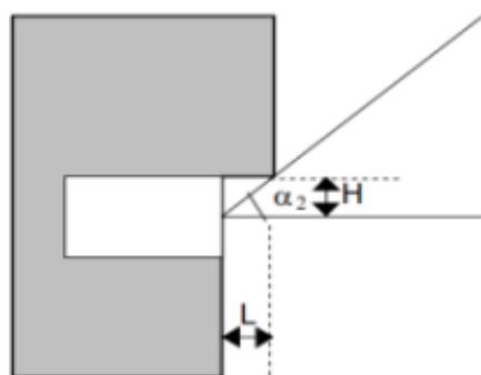
Figura 2 Valore del fattore finestra \varepsilon per ostruzioni superiori
