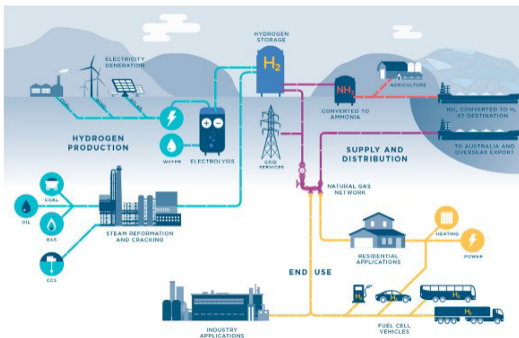
Figura 3 Schema della filiera dell'idrogeno. Fonte: Powermagazine 9
