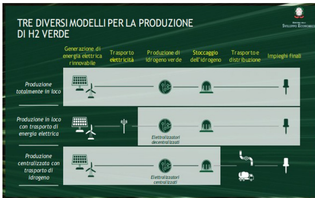
Figura 8 Produzione, trasporto e stoccaggio di H2 verde.
