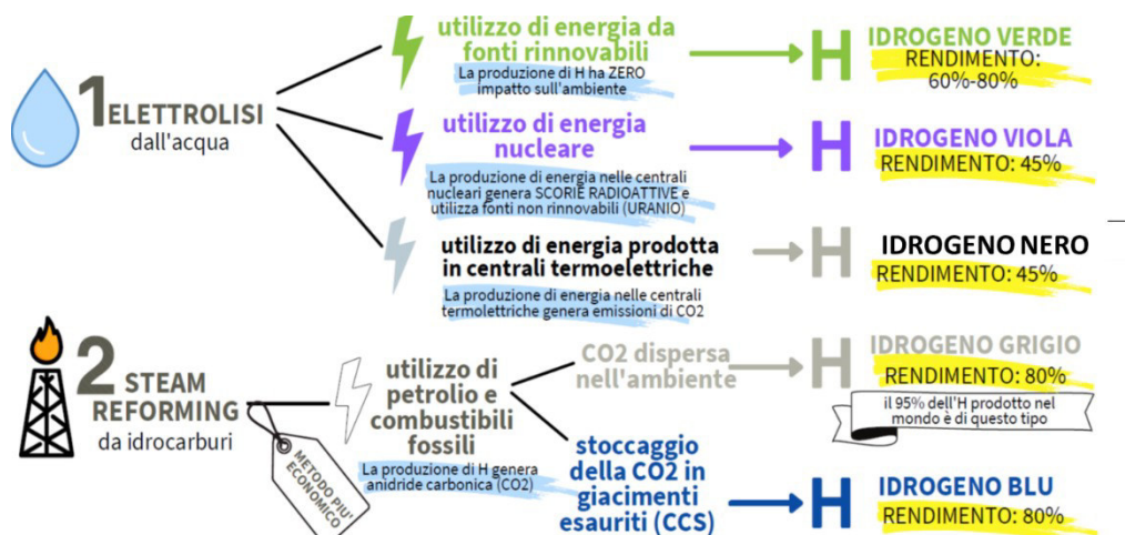
Figura 1 Schematizzazione della produzione di idrogeno, i suoi impatti ambientali e i suoi rendimenti.
